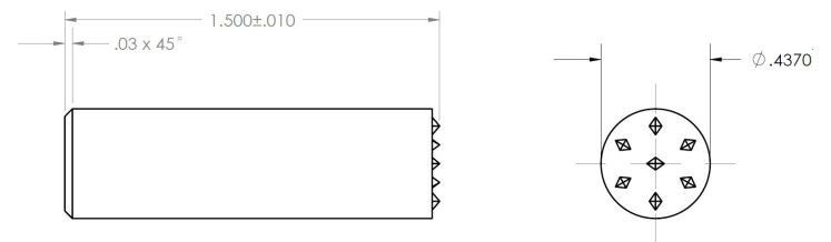
Dimensiones TruGARD SD
